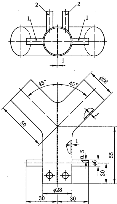
图 4 口具组件式呼吸器试验用连接器
