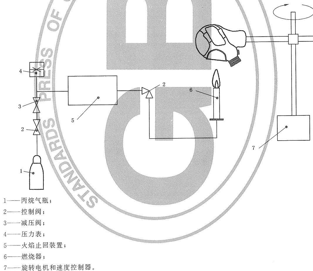
图 6 可燃性检测装置示意图
